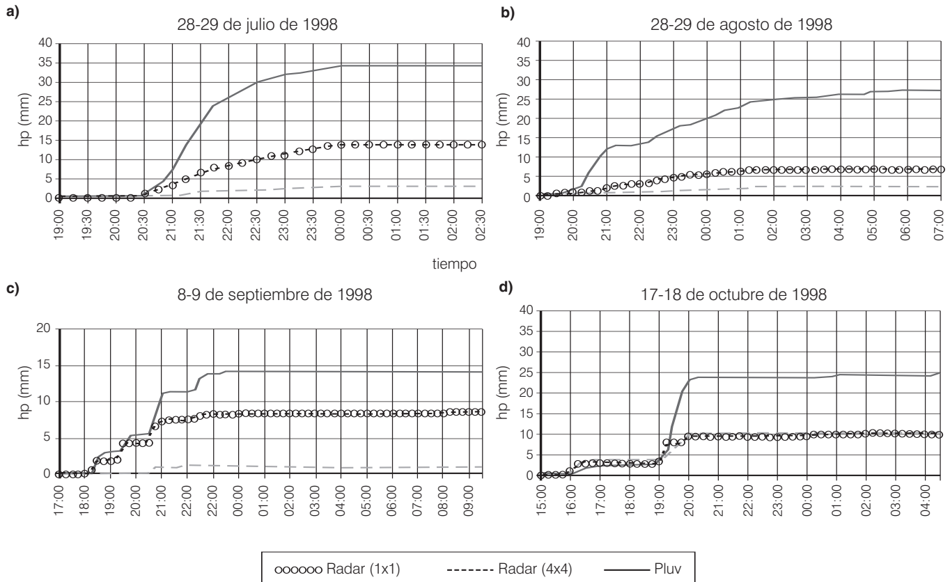
Ilustración 6. Comparación de lluvias estimadas: con pixeles de 1x1 km, con pixeles de 4x4 km y con pluviógrafos.
