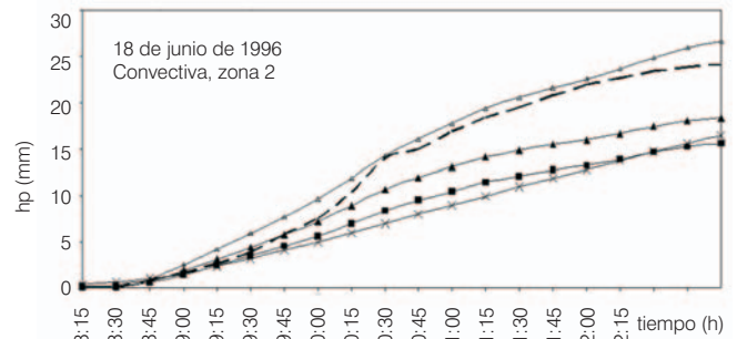
Ilustración 12. Curvas masa de cada una de las tormentas estimadas con pluviógrafos, Marshall-Palmer y ajuste.
