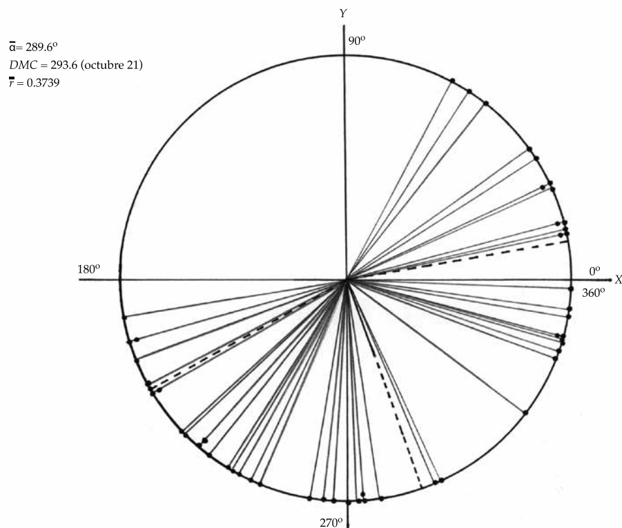
Figura 2. Representación de las fechas de ocurrencia y de los índices de estacionalidad de las crecientes anuales de la estación hidrométrica Huites de la Región Hidrológica 10 (Sinaloa).
