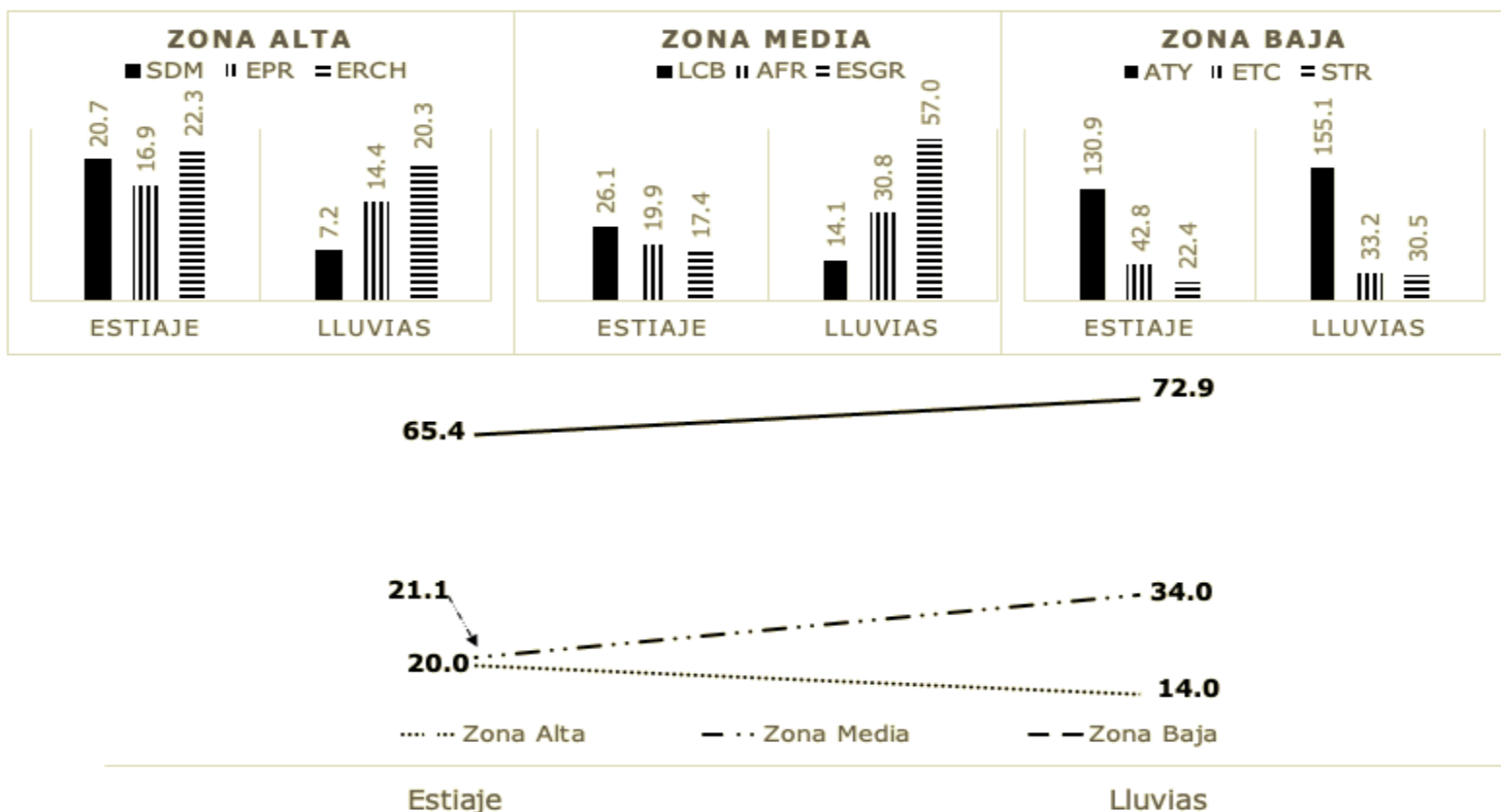
Figura 11. DBO 5 promedio en las zonas alta, media y baja del río Atoyac, Guerrero, durante las épocas de estiaje y lluvia.
