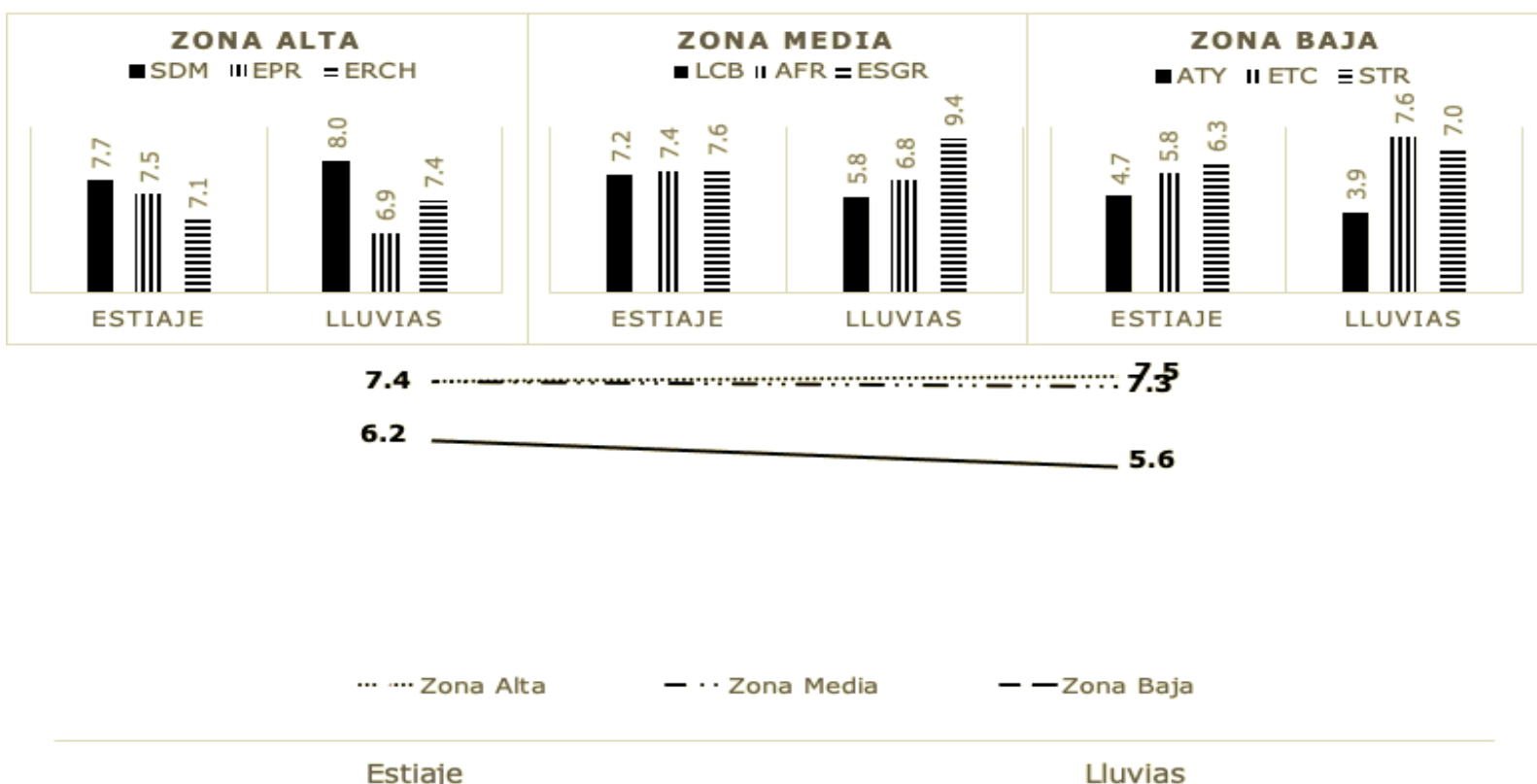
Figura 10. OD promedio en las zonas alta, media y baja del río Atoyac, Guerrero, durante las épocas de estiaje y lluvia.
