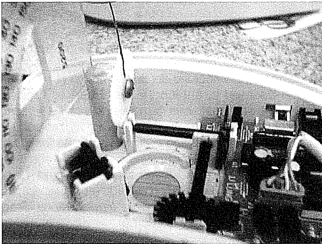
Ilustración 4. Diagrama del dispositivo propuesto para medir la velocidad de un fluido utilizando el "ratón" de una computadora.
