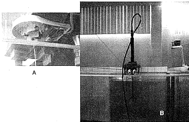
Ilustración 8. Fotografía del dispositivo y el correntímetro acústico (ADV) utilizado para las pruebas en agua.
